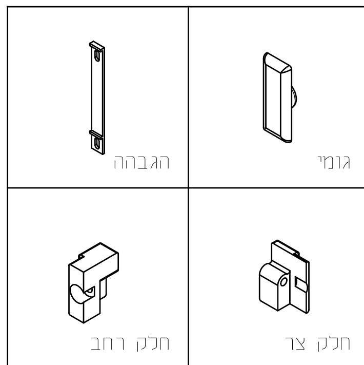
4. הכנסת החלק הרחב של הבולם מעל החלק הצר
