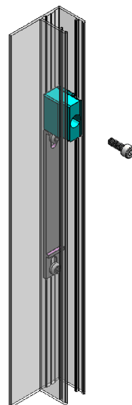
5. הורדת החלק הרחב על החלק הצר ותפיסתו בעזרת בורג
