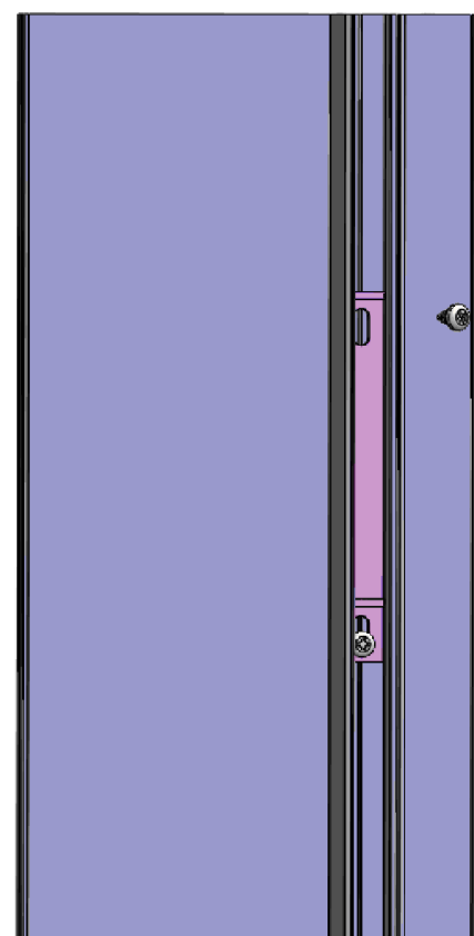
2. חיבור ההגבהה עם ברגים
