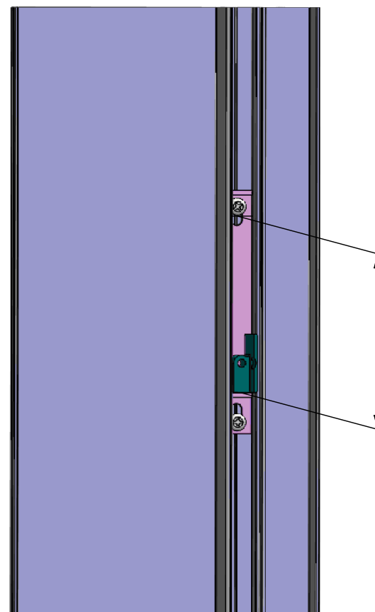
3. הכנסת החלק הצר של הבולם בין הבורג העליון למדרגה
