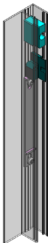
4. הכנסת החלק הרחב של הבולם מעל החלק הצר
