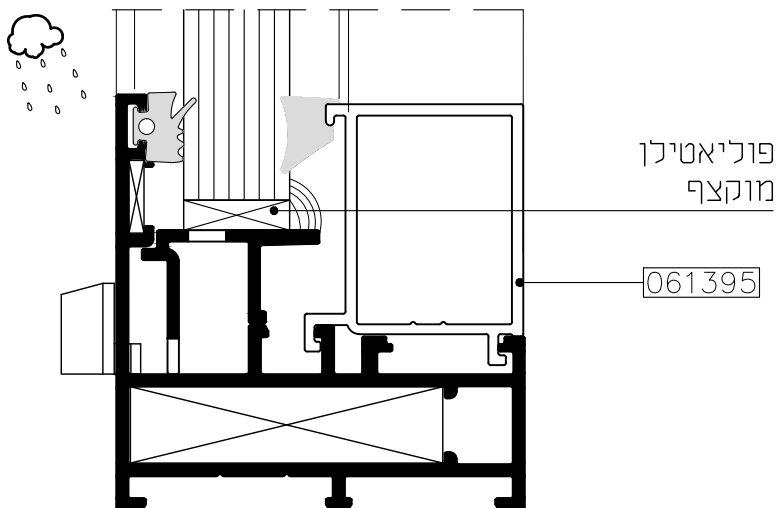
זכוכית 14 מ"מ
