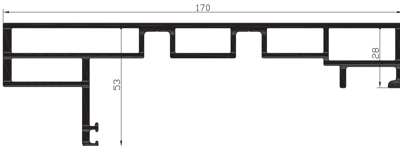
פרופיל עליון לחתון לרפפה
