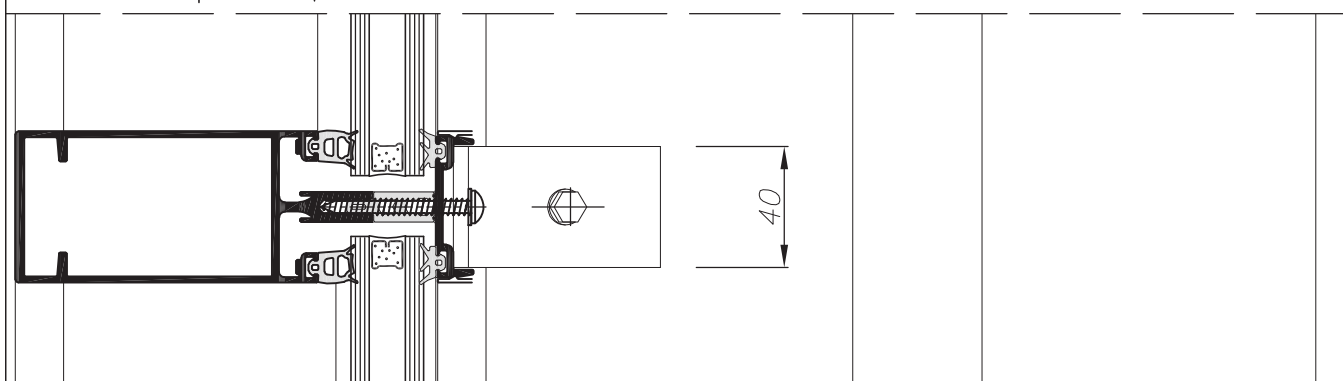
חתך A-A קנ"מ 1:2.5
