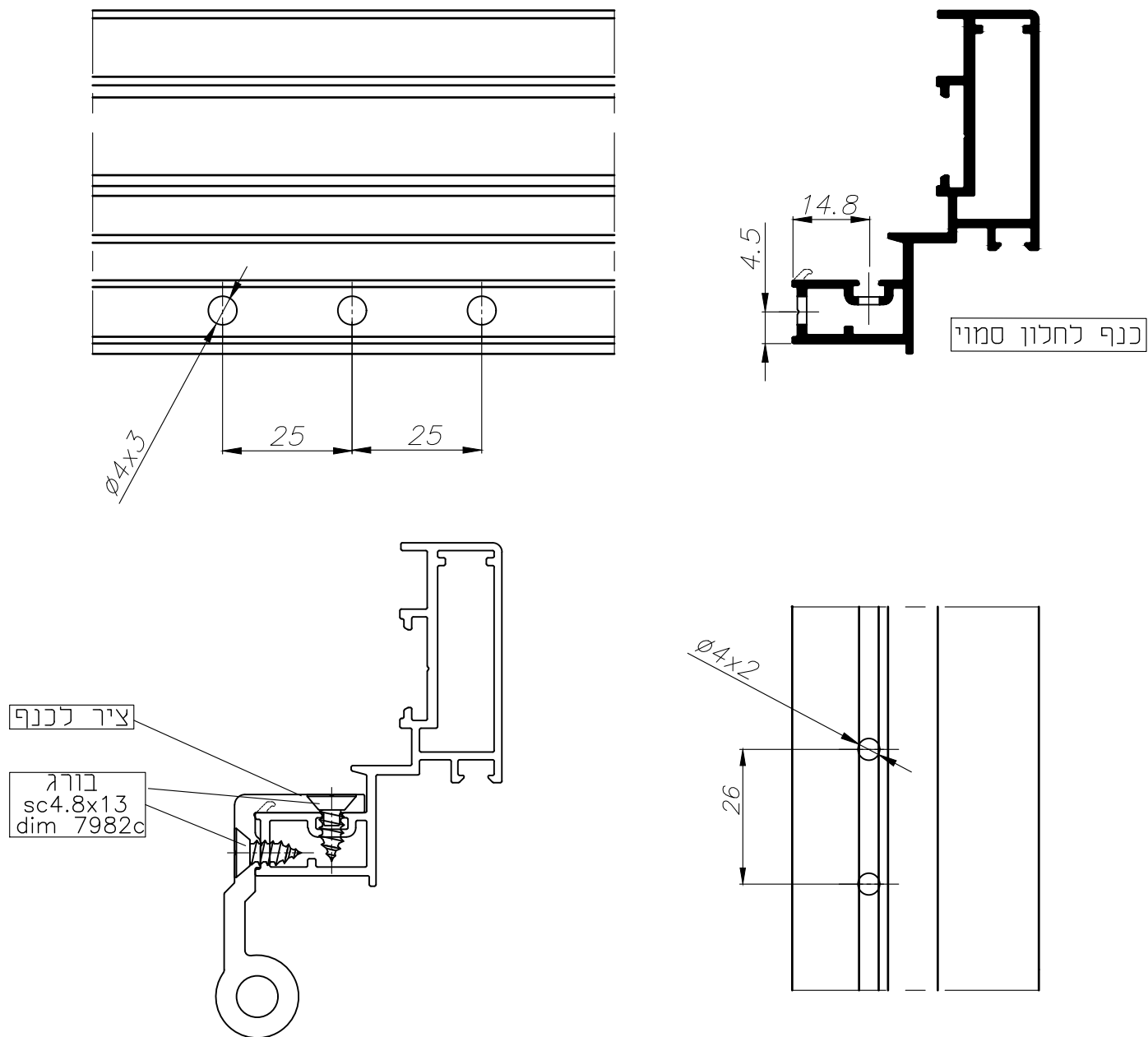
עיבוד פרופיל-חלק עליון של ציר מילוט
