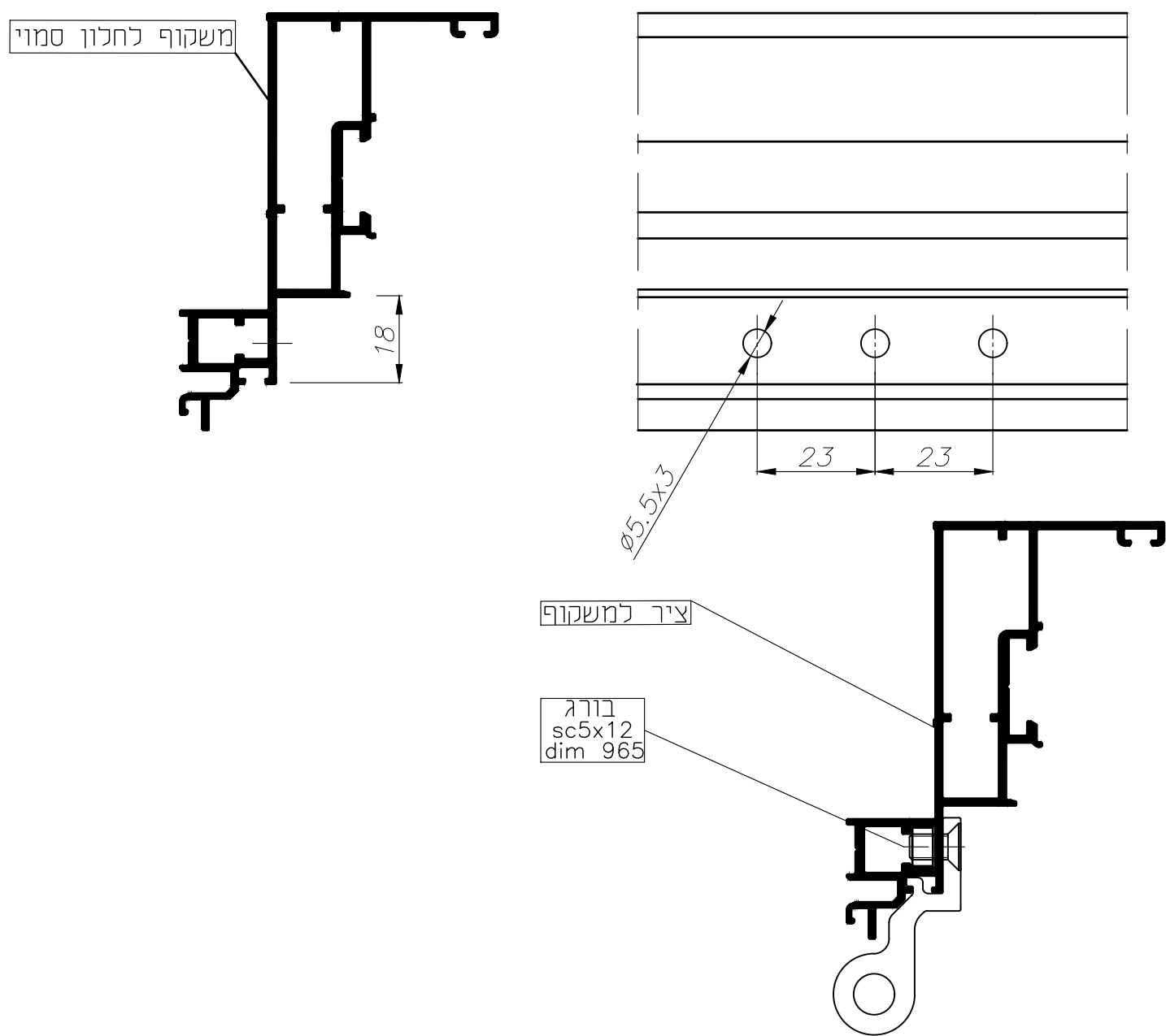
עיבוד פרופיל-חלק תחתון של ציר מילוט
