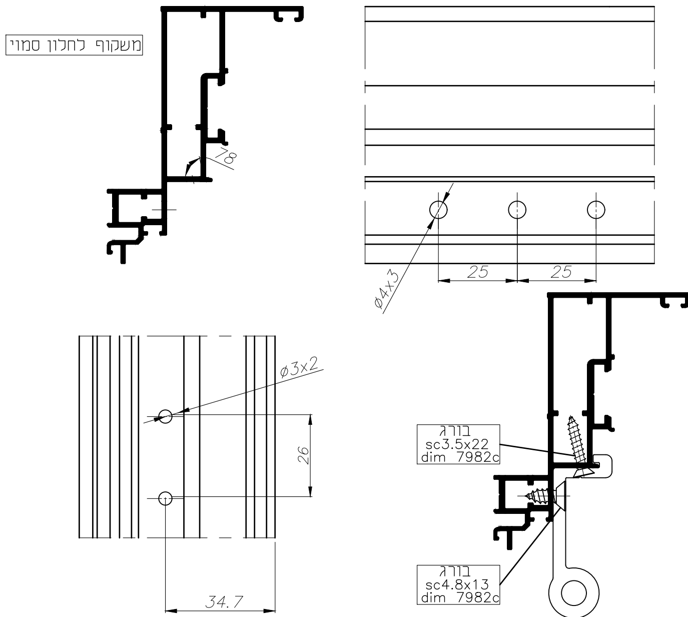
עיבוד פרופיל-חלק תחתון של ציר מילוט
