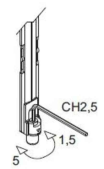
כיוונון בריח
