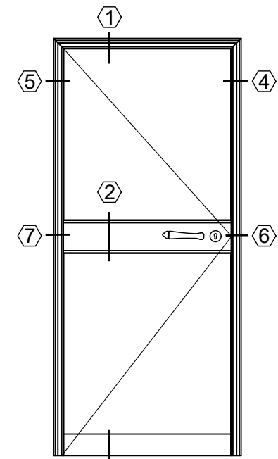
מידות מירביות לכנף דלת 90cmX210cm
