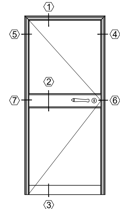
מידות מירביות לכנף דלת 90cmX210cm
