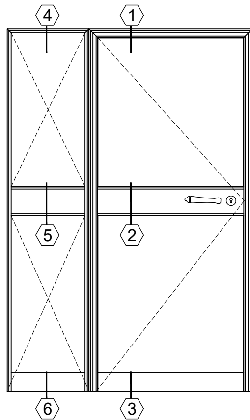
מידות מירביות לכנף דלת 90cmX210cm
