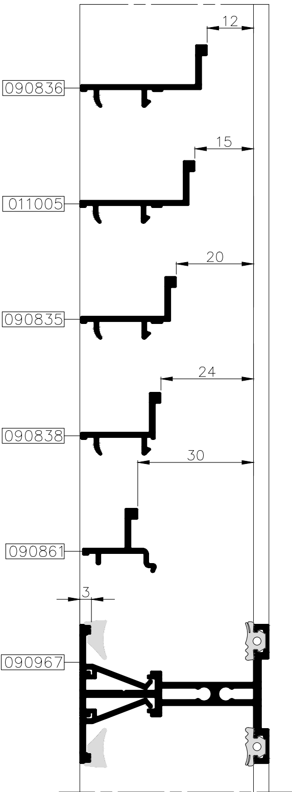
סרגל נמוך
