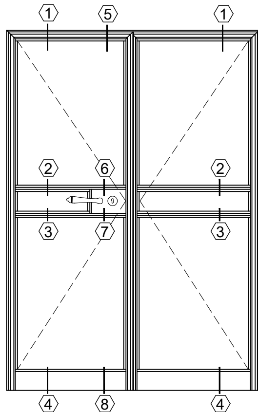
מידות מירביות לכנף דלת 90cmX210cm
