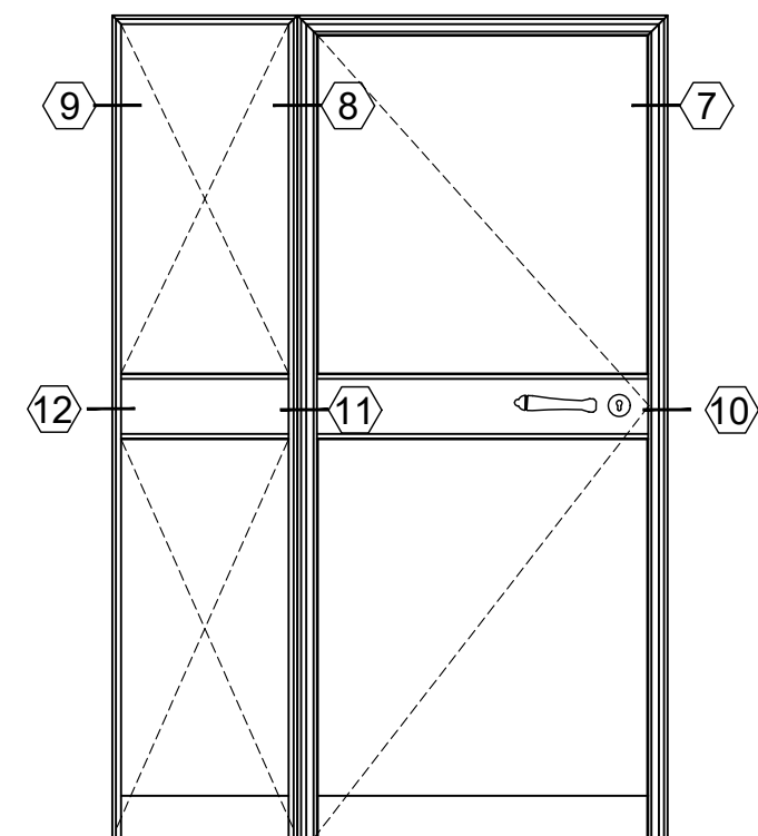
מידות מירביות לכנף דלת 90cmX210cm
