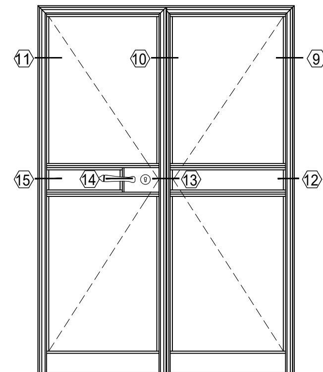
מידות מירביות לכנף דלת 90cmX210cm
