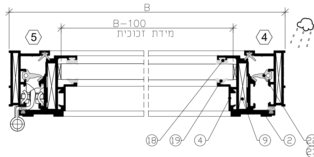
מידות מירביות לכנף דלת 90cmX210cm
