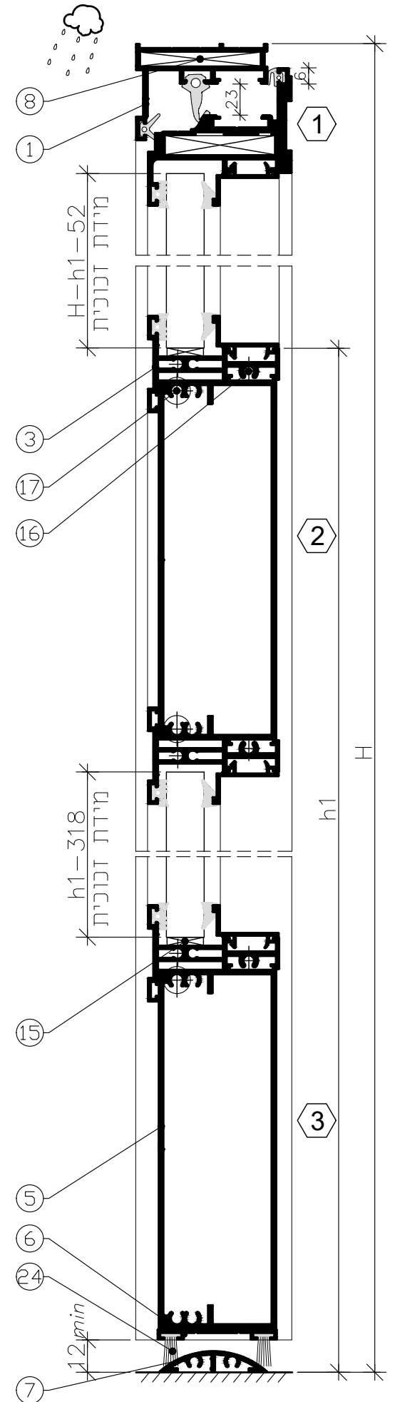
מידות מירביות לכנף דלת 90cmX210cm
