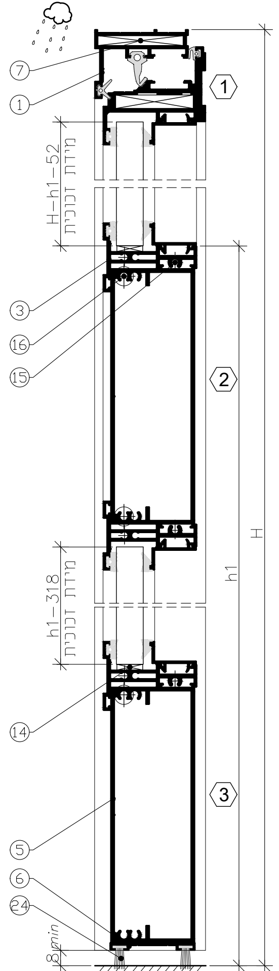
מידות מירביות לכנף דלת 90cmX210cm
