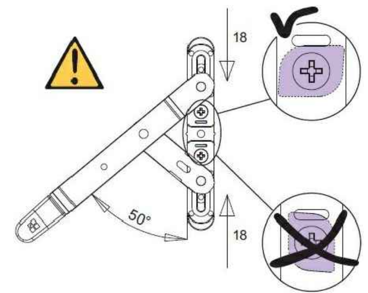
הרכבת פרפר
