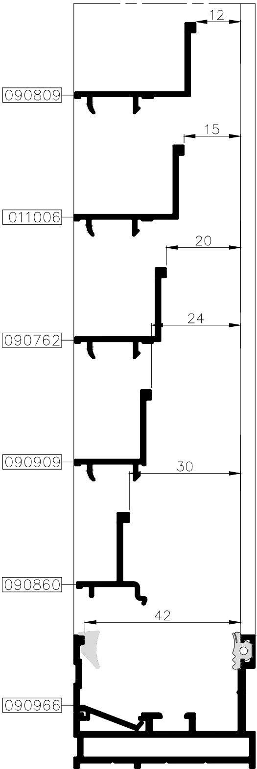
סרגל גבוה
