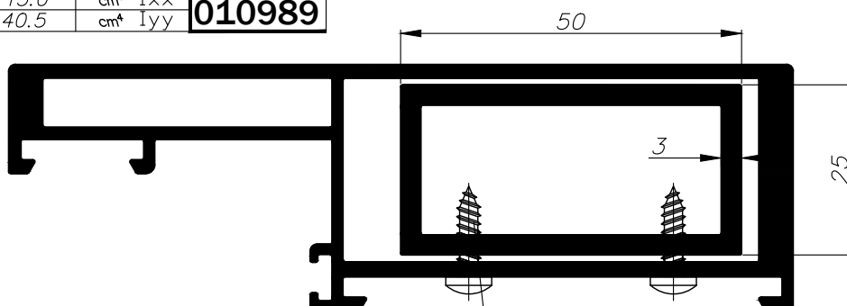
אלמנט חידוק מהודק למאחז היד ע"י ברגים ST 3.5*19 DIN7981 כל 50 ס"מ
